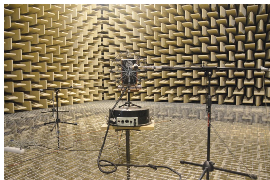
Bezdozvuková komora pro akustická měření na katedře fyziky Elektrotechnické fakulty ČVUT.
